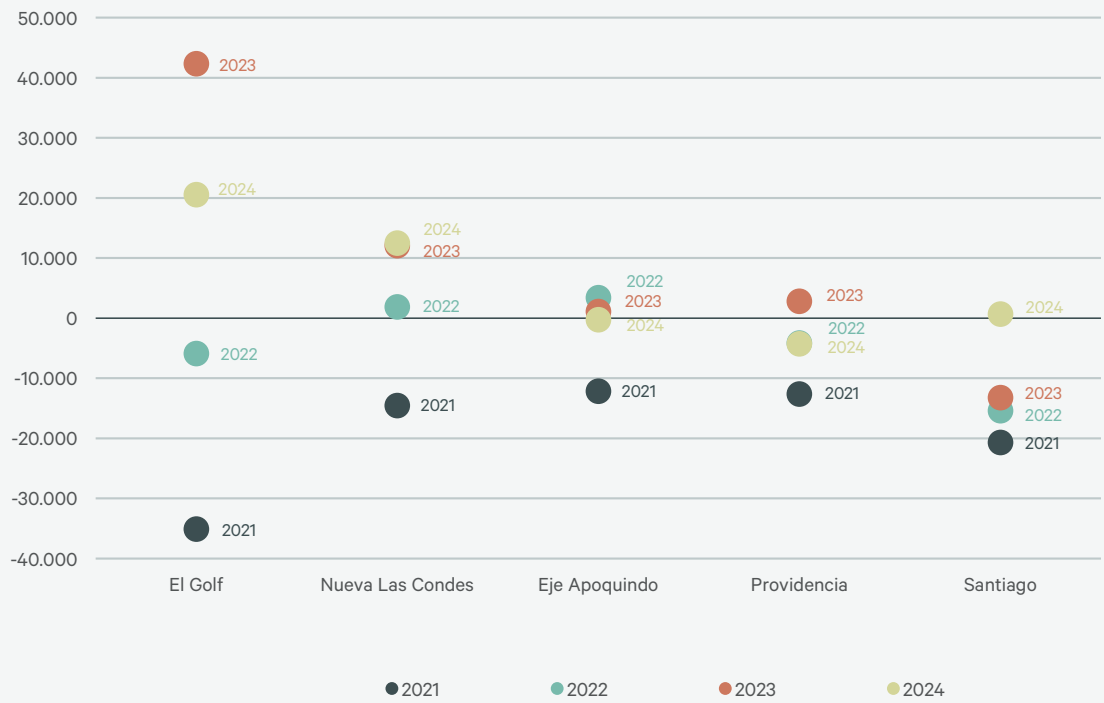
FIGURA 9 Absorción Neta Año Móvil Clase A (m²)
